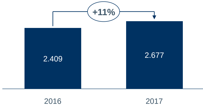
राजस्व (€m)
