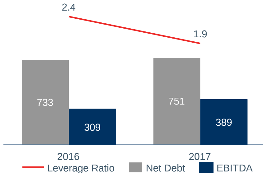
उत्तोलन (€m)
